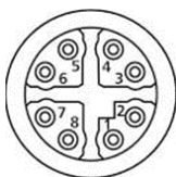
X-coding
