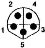
B-coding
